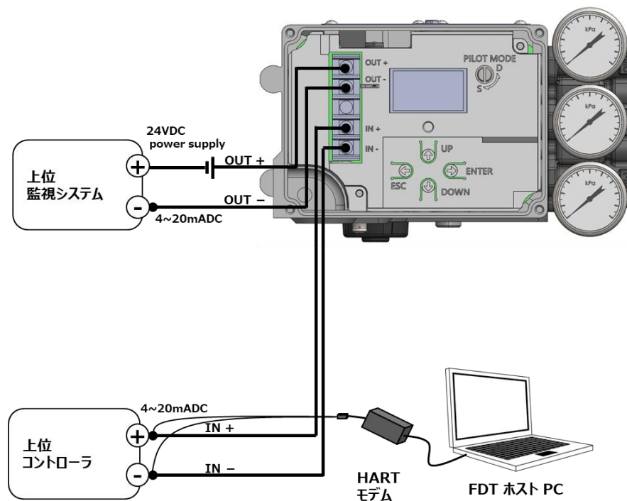
図 1.4d ケーブル 2 本(2 芯)による電気配線
