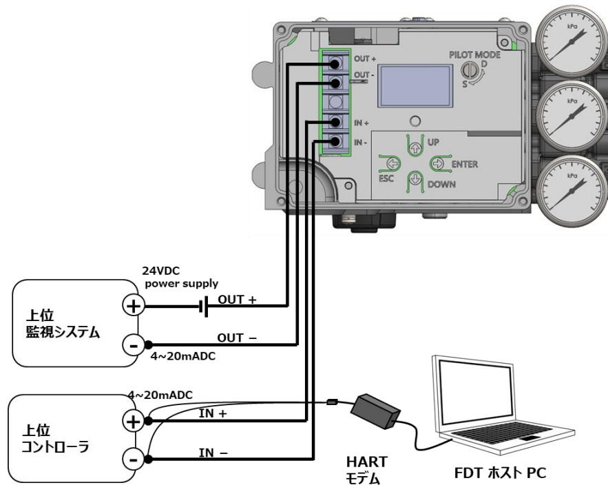
図 1.4c ケーブル 1 本(4 芯)による電気配線
