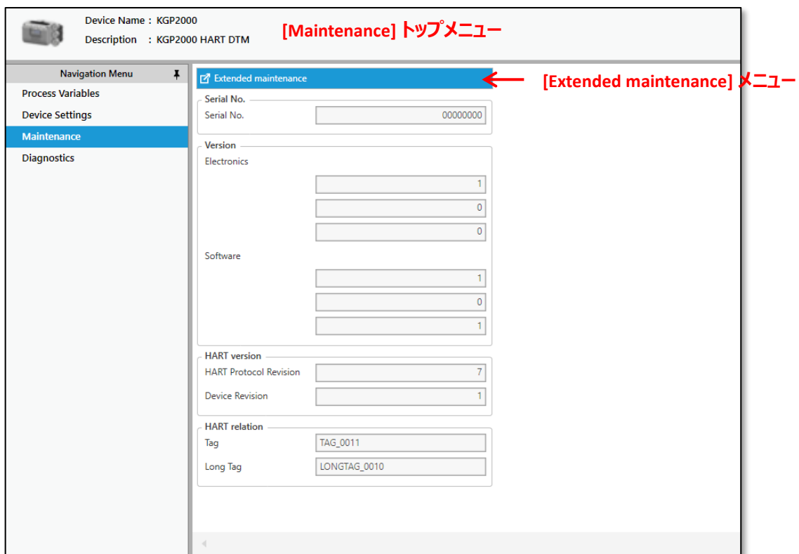
図 2.2.3a [Maintenance]トップメニュー
