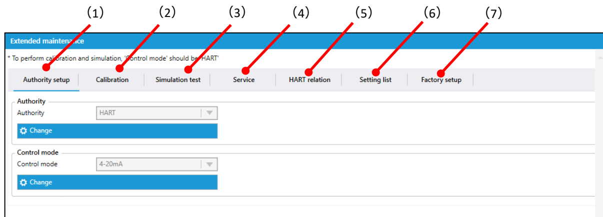
図 2.2.3b [Extended maintenance] メニュー
